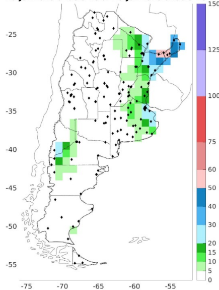
Pronóstico de precipitación acumulada (mm) del 20-Jul-2019 a las 9 hs al 26-Jul-2019 a las 9 hs
